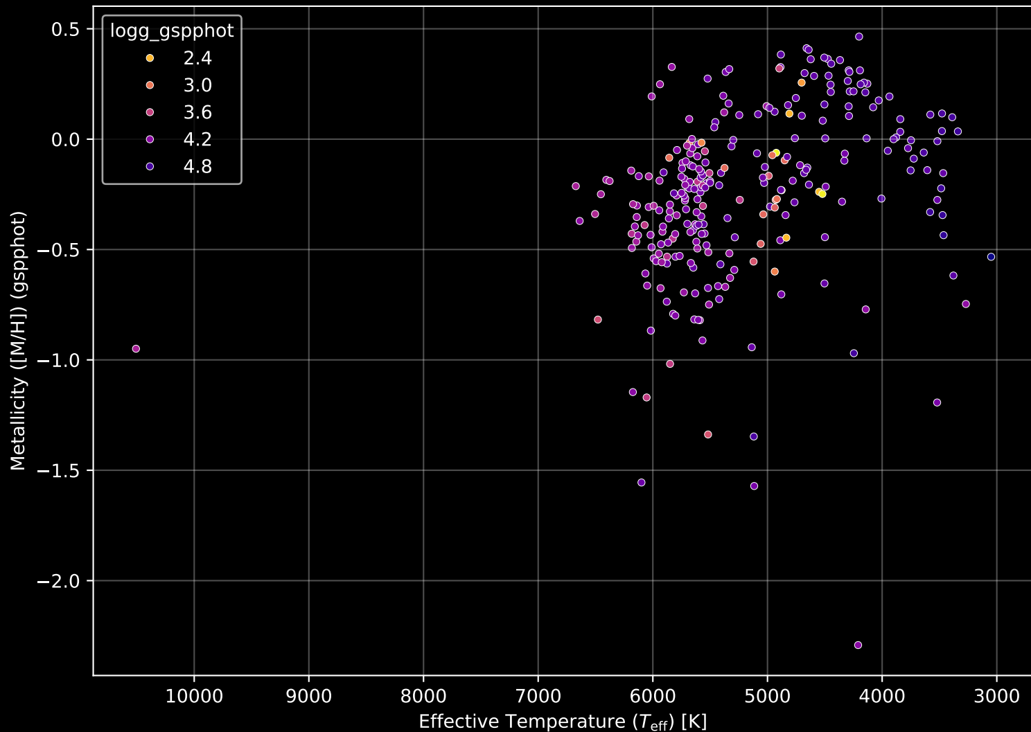
APOGEE DR17 Field: [sgr_tidal7] Stellar Population Parameters (n= 273)
